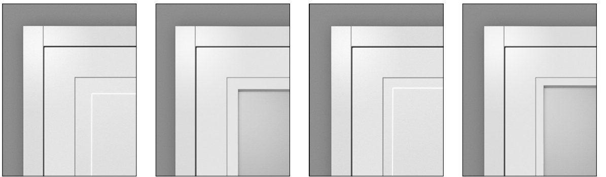
OT.60 – das Profil (60 mm) OT.60 – die Glasleiste (40 mm) OT.40 – das Profil (40 mm) OT.40 – die Glasleiste (25 mm)
